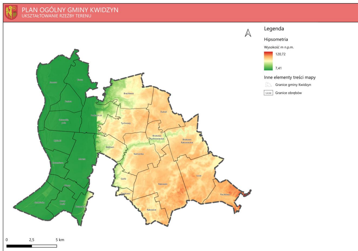
Ryc. 7. Ukształtowanie rzeźby terenu w gminie Kwidzyn
