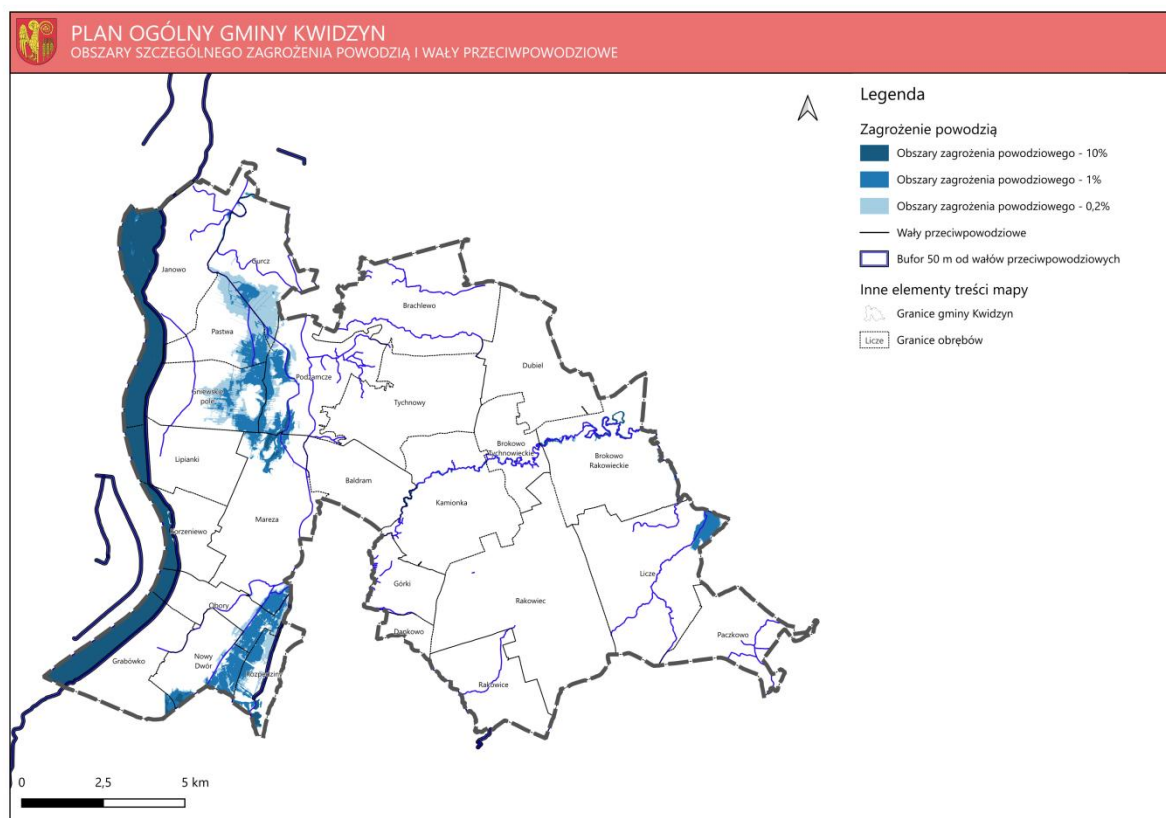
Ryc. 17. Mapa zagrożenia powodziowego z prawdopodobieństwem wystąpienia 10%, 1%, 0,2%
